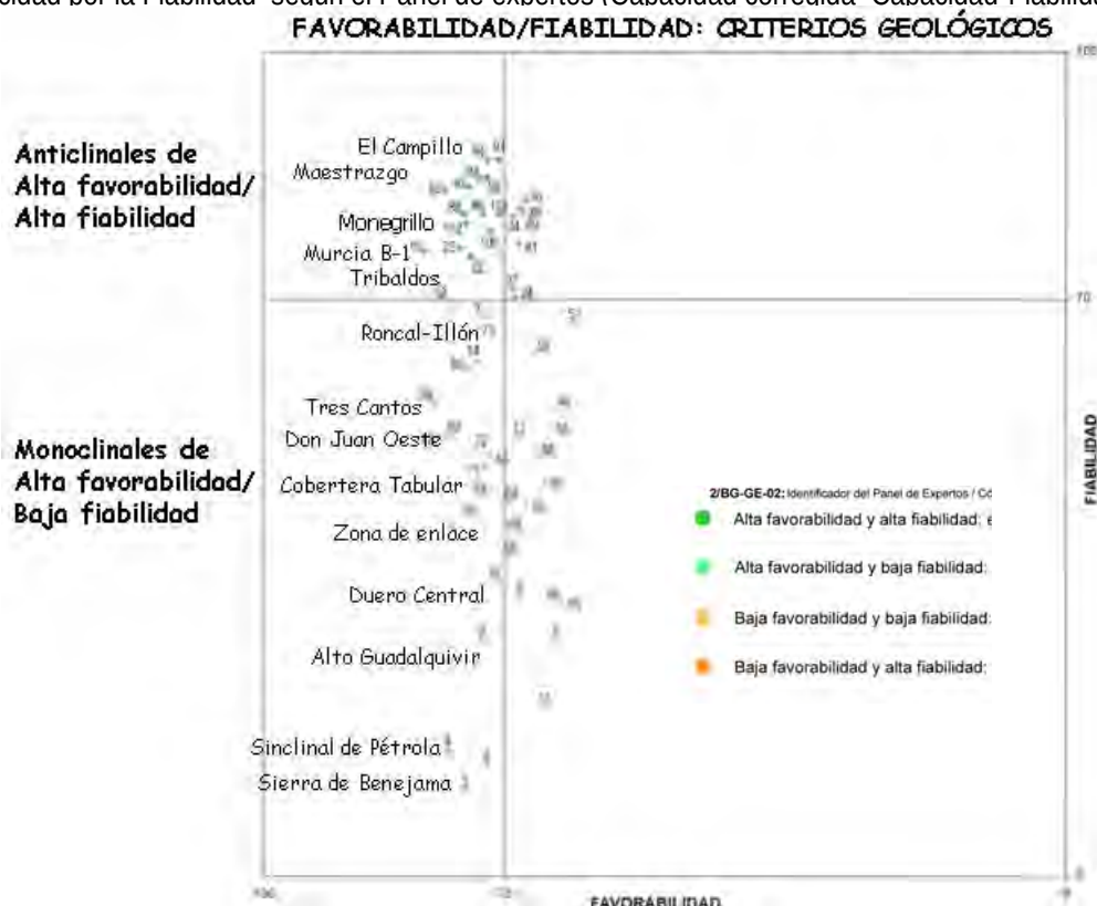
Figura 15. Estructuras geológicas según Favorabilidad / Fiabilidad en geología (Fuente: Panel Expertos)
