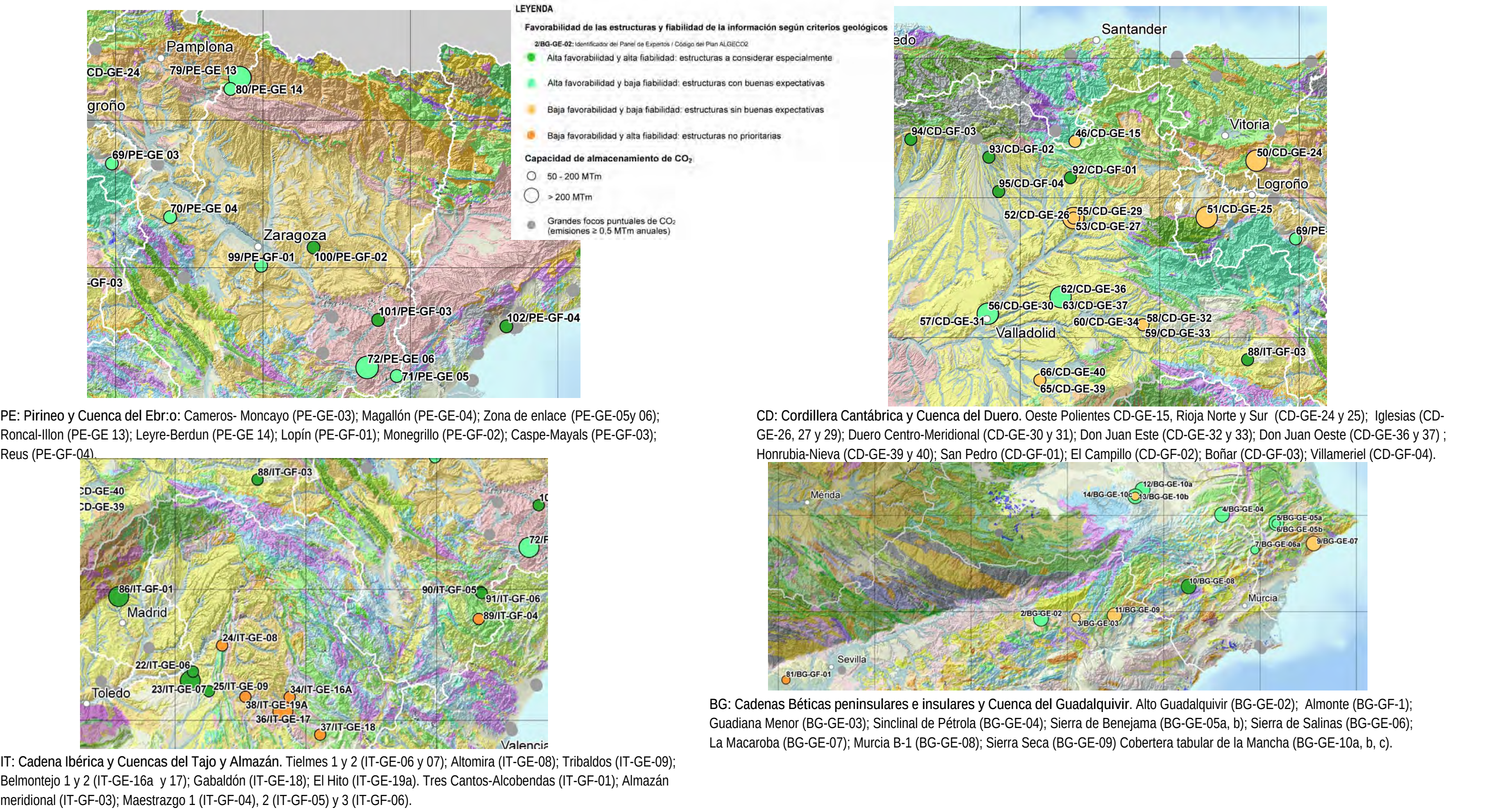
Figura 10. DETALLES DE MAPAS DE FAVORABILIDAD/FIABILIDAD DE LAS ESTRUCTURAS GEOLÓGICAS ESTUDIADAS. Favorabilidad según Criterios geológicos. 55 Almacenes de capacidad superior a los 50 Mt CO 2 . PE: 10 estructuras; CD: 19 estructuras; IT: 13 estructuras; BG: 13 estructuras. Base: mapa geológico de España 1: 1.000.000.
